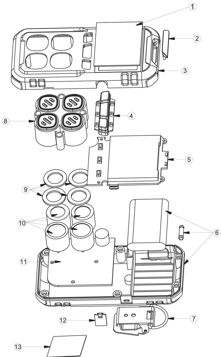
Рисунок 14 - Схема запасных частей
